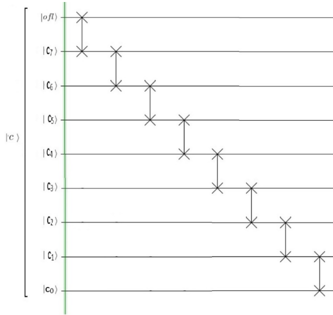
شکل ۱۰ مدار ضرب در دو پیاده‌سازی شده با شیفت به چپ
